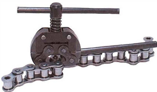
Extractor de eje de cadenas réf 16913050 Cadenas simples, dobles, triples al paso de 6.35 a 19,05mm ISO & ASA
